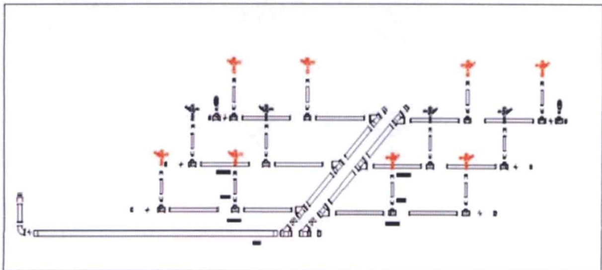
Figura 02. Representação do sistema hidráulico na área de rustificação
